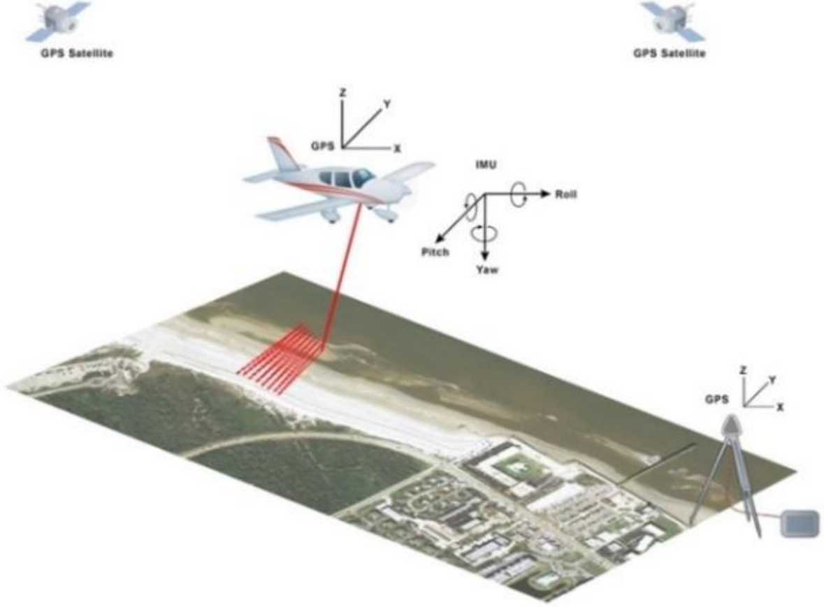
Şekil 1. Hava LiDAR sistemi (URL 1)
